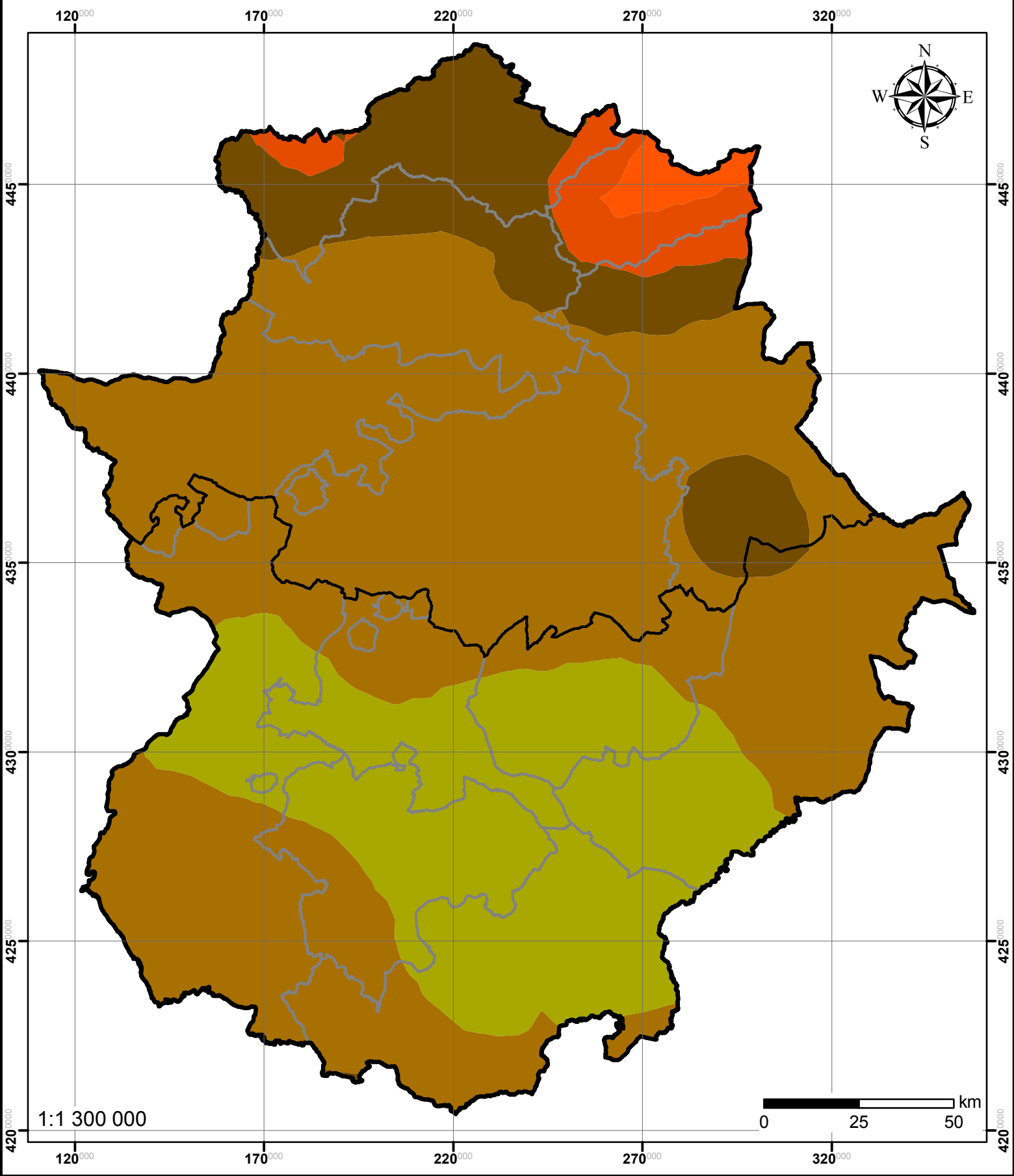
Mapa 62. Variación de la precipitación acumulada anual promedio del periodo 2041-2070 (Escenario A2) respecto del promedio del periodo 1961-1990.
