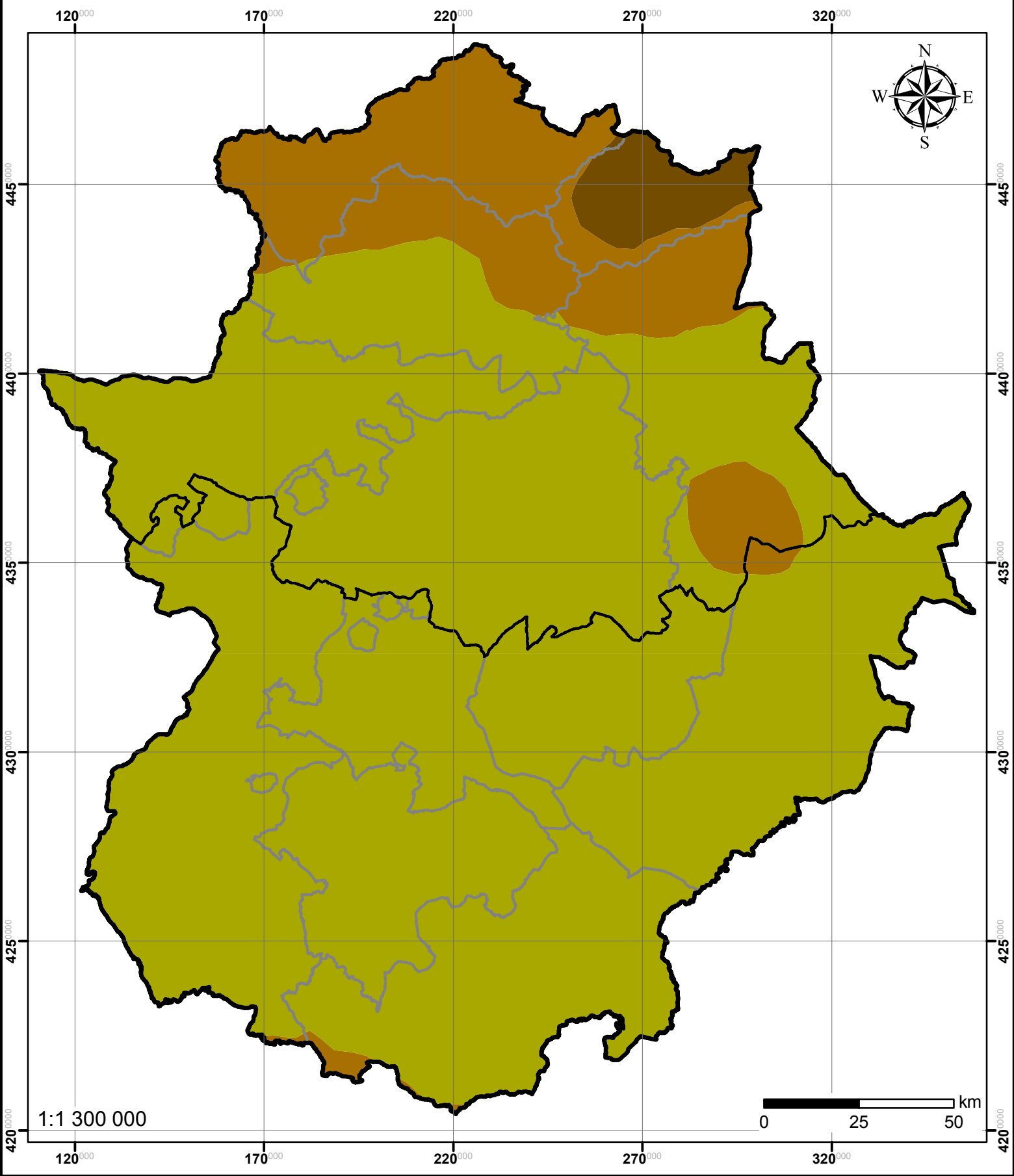
Mapa 60. Variación de la precipitación acumulada anual promedio del periodo 2011-2040 (Escenario A2) respecto del promedio del periodo 1961-1990.
