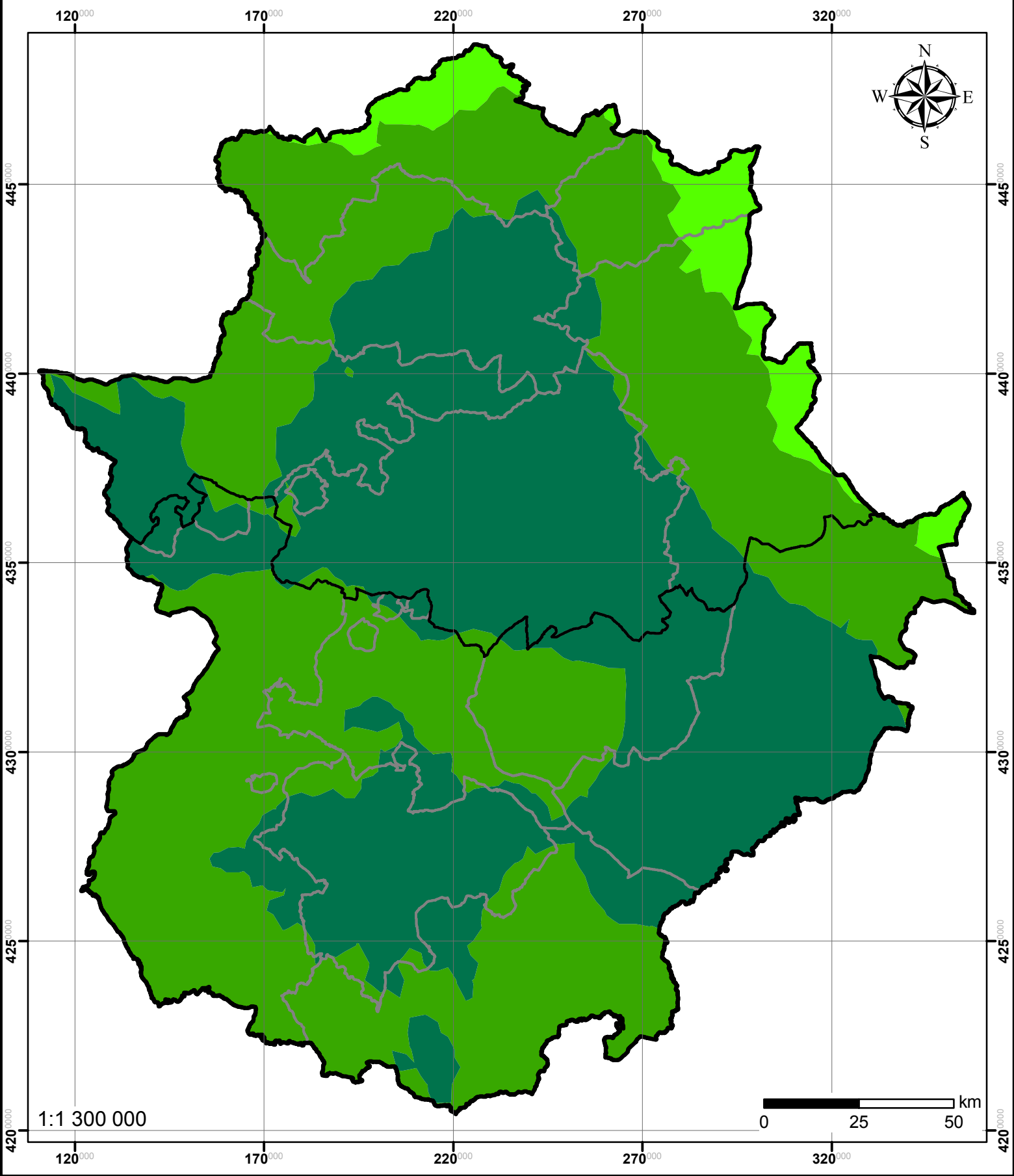
Mapa 42. Temperatura media anual de las mínimas diarias del promedio 2041-2070. Escenario A2.
