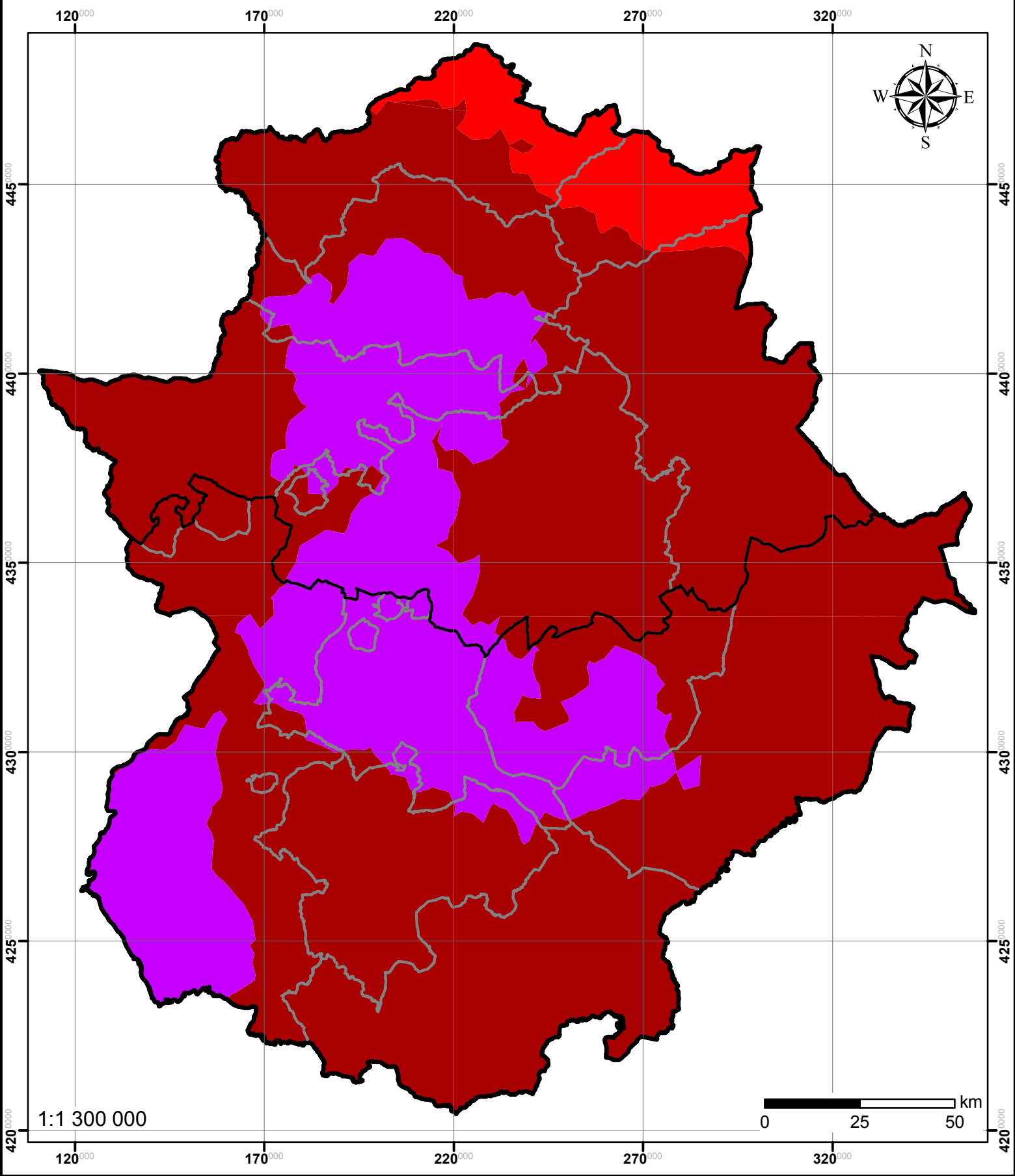
Mapa 39. Temperatura media anual de las máximas diarias del promedio 2041-2070. Escenario B2.
