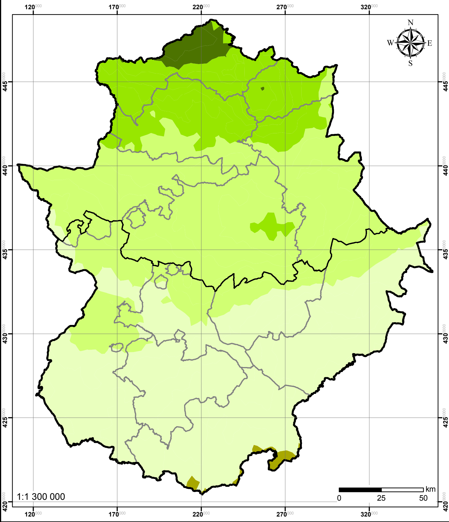
Mapa 33. Variación de la precipitación acumulada anual en el año 2050 (Escenario B2) respecto del promedio del periodo 1961-1990.
