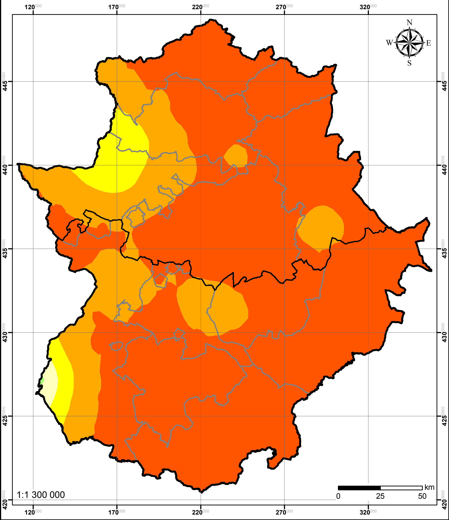
Mapa 21. Aumento de la temperatura media anual de las máximas diarias en el año 2050 (Escenario B2) respecto del promedio del periodo 1961-1990.
