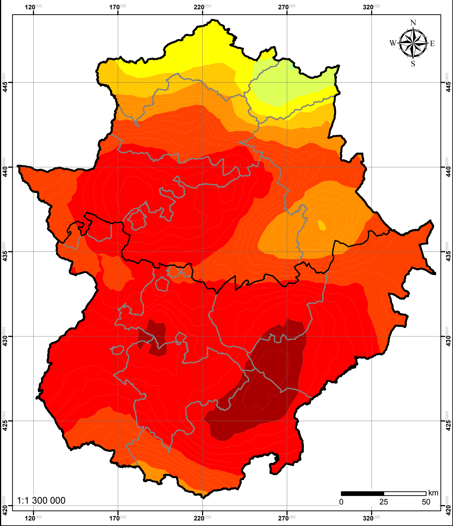
Mapa 16. Precipitación acumulada anual promedio del año 2050. Escenario A2.
