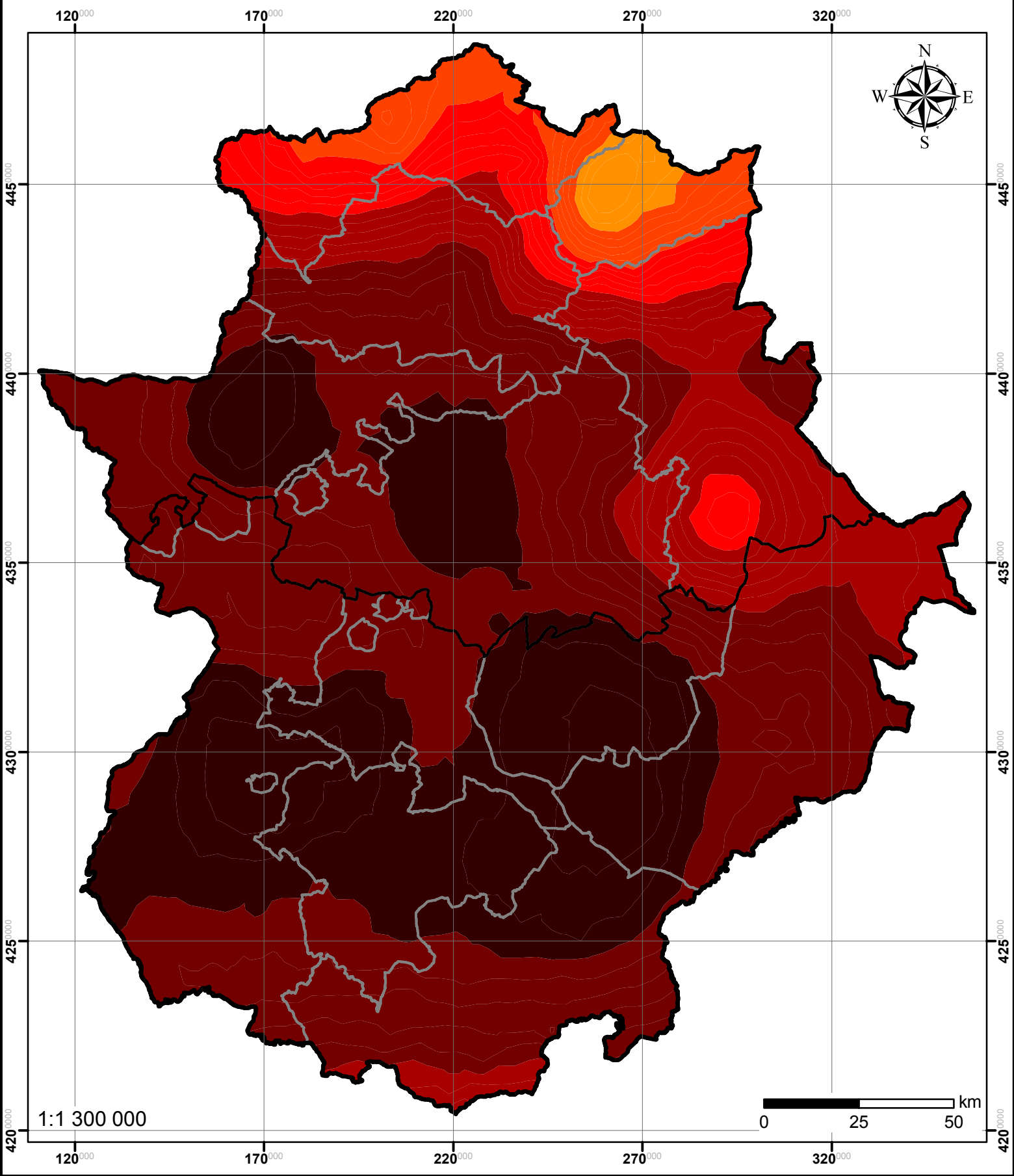
Mapa 15. Precipitación acumulada anual promedio del año 2025. Escenario B2.
