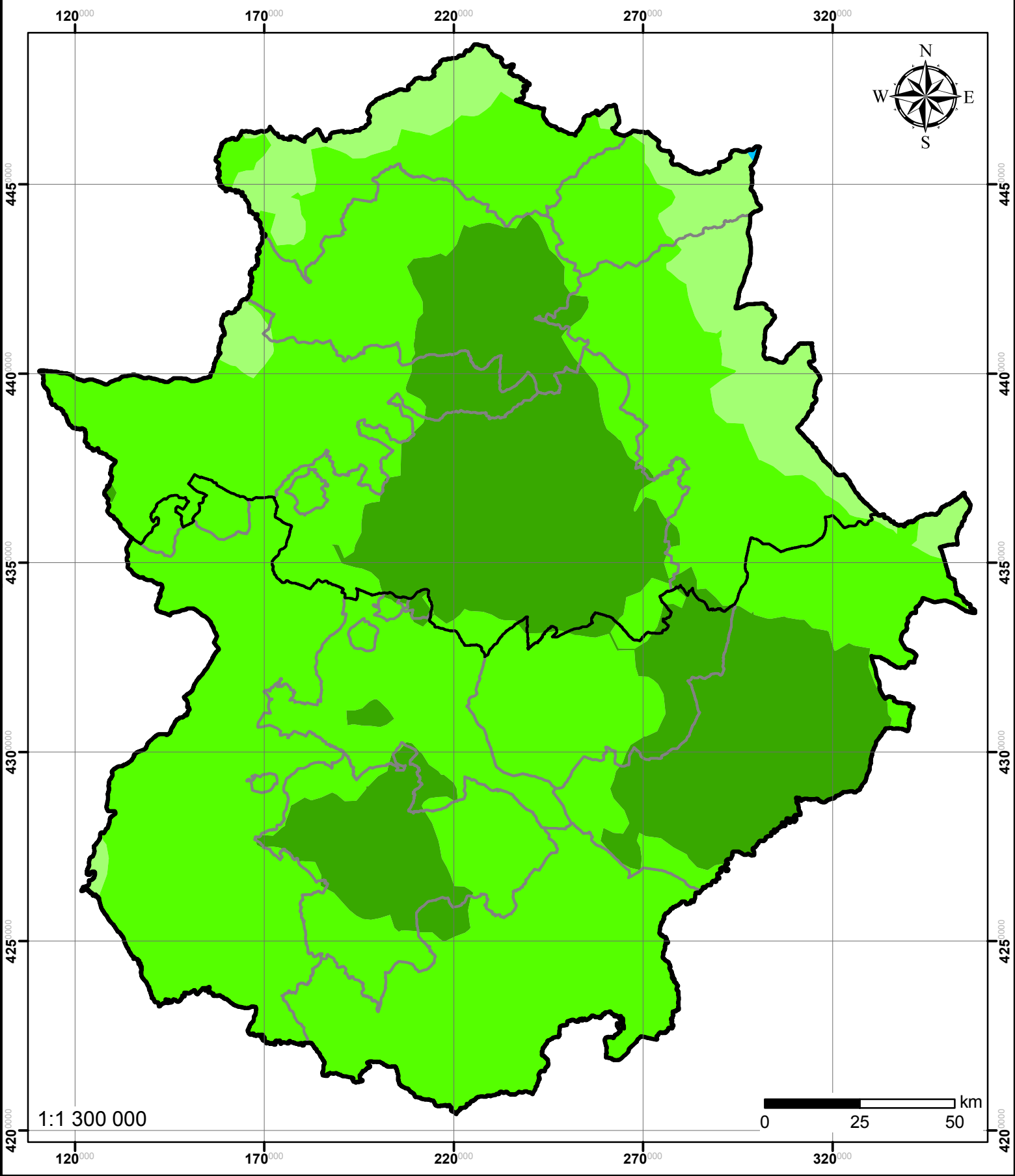
Mapa 12. Temperatura media anual de las mínimas diarias del año 2050. Escenario B2.
