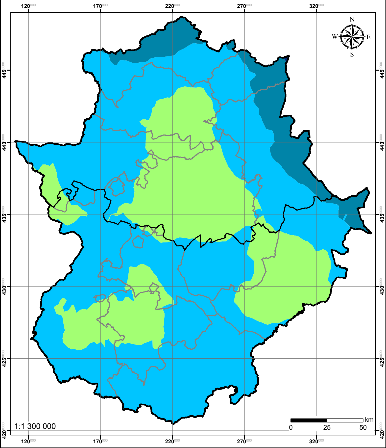
Mapa 8. Temperatura media anual de las mínimas diarias del promedio 1961-1990.
